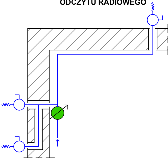
RYS.3. TRZY PUNKTY CZERPALNE JEDEN PODLICZNIK INSTALACJA WODOCIĄGOWA PROWADZONA W ŚCIANIE/POSADZCE WODMIERZ Z NAKŁADKĄ DO ODCZYTU RADIOWEGO
