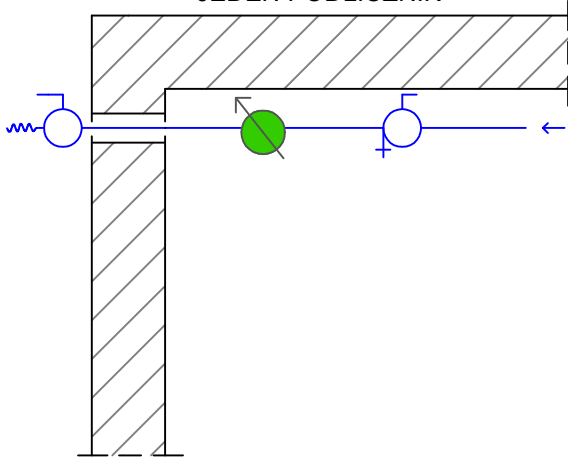
RYS.3. TRZY PUNKTY CZERPALNE JEDEN PODLICZNIK INSTALACJA WODOCIĄGOWA PROWADZONA W ŚCIANIE/POSADZCE WODMIERZ Z NAKŁADKĄ DO ODCZYTU RADIOWEGO
