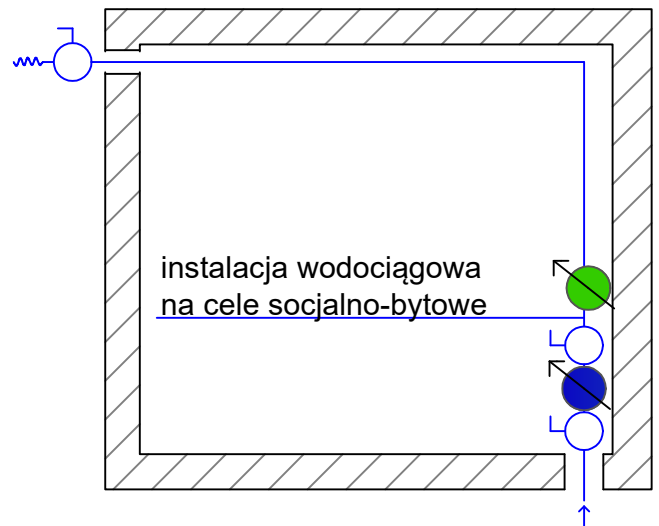
RYS.4. LOKALIZACJA POLICZNIKA BEZPOŚREDNIO ZA ZESTAWEM Z WODMIERZEM GŁÓWNYM WODMIERZ Z NAKŁADKĄ DO ODCZYTU RADIOWEGO
